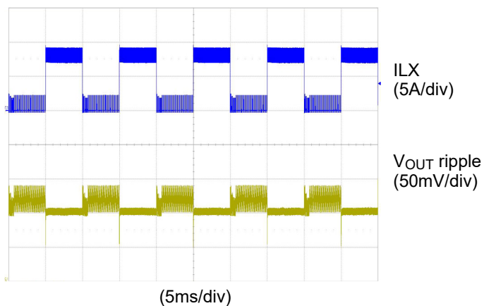
Load Transient 0A to 8A
