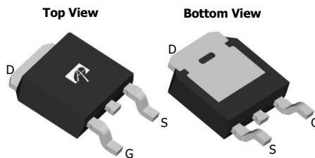
TO252 DPAK
